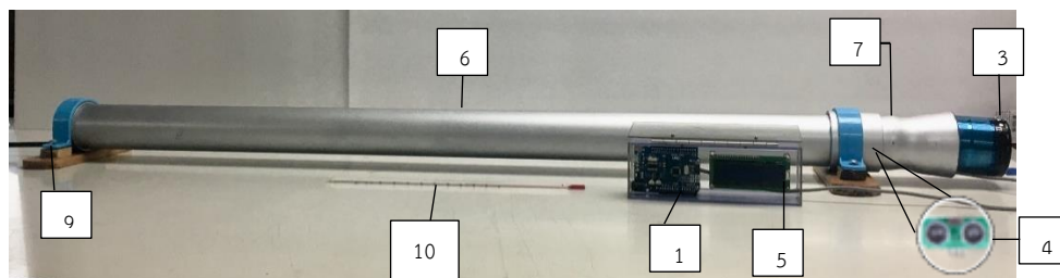
ภาพที่ 1 ชุดการทดลอง เรื่อง การสั่นพ้องของคลื่นเสียงในท่อโดยใช้ Arduino
